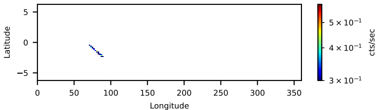
60861003003: 30 to 120 keV
