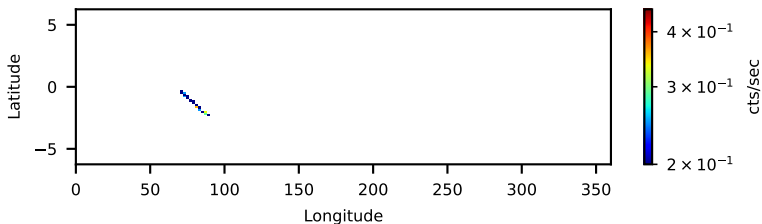
60861003003: 3 to 10 keV
