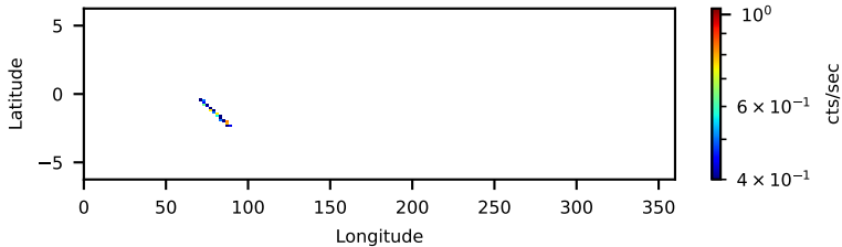
60861003003: 3 to 120 keV
