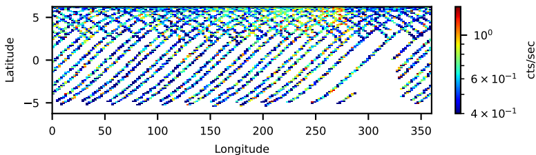
60861002002: 3 to 120 keV
