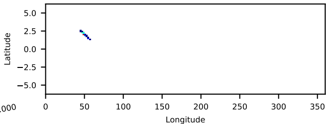
60860010001: 3 to 10 keV
