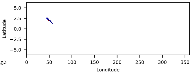
60860010001: 30 to 120 keV
