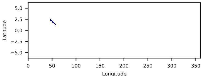
60860010001: 30 to 120 keV
