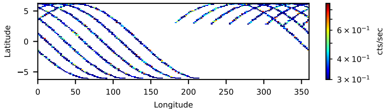
60802039006: 30 to 120 keV
