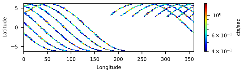
60802039006: 3 to 120 keV
