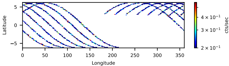
60802039006: 3 to 10 keV
