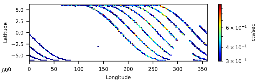
60802038006: 30 to 120 keV
