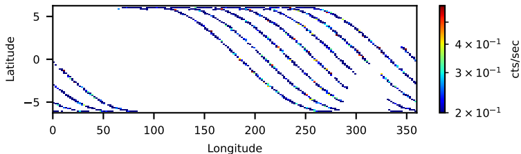
60802038006: 3 to 10 keV
