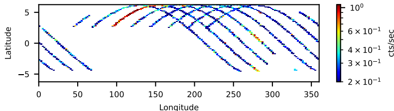
60802036006: 3 to 10 keV
