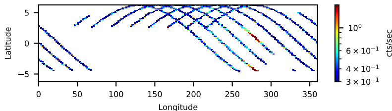
60802036006: 30 to 120 keV
