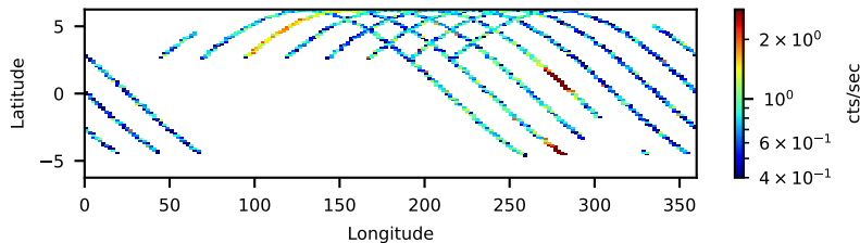
60802036006: 3 to 120 keV
