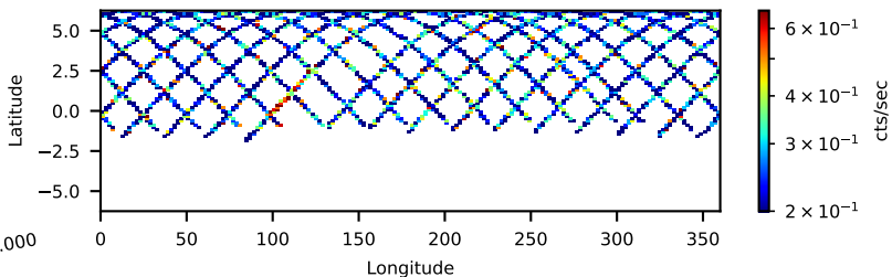
60802036002: 30 to 120 keV
