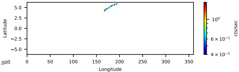
60802036001: 3 to 10 keV
