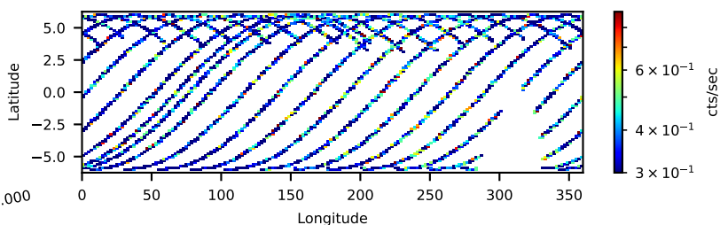
60802019006: 30 to 120 keV
