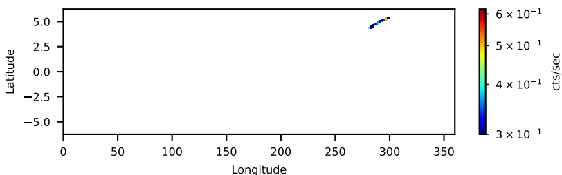
60802019003: 30 to 120 keV
