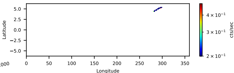
60802019003: 3 to 10 keV
