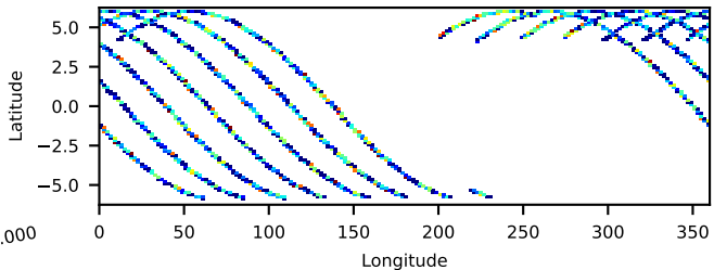
60802014006: 3 to 10 keV
