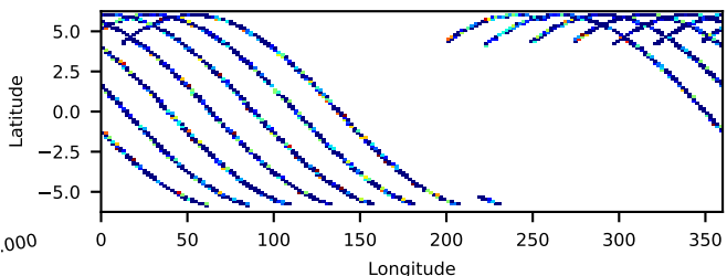
60802014006: 30 to 120 keV
