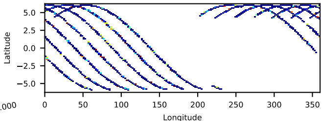
60802014006: 30 to 120 keV
