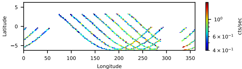
60802013004: 3 to 120 keV
