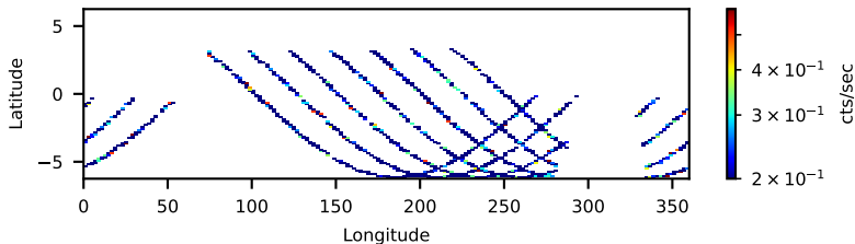
60802013004: 3 to 10 keV
