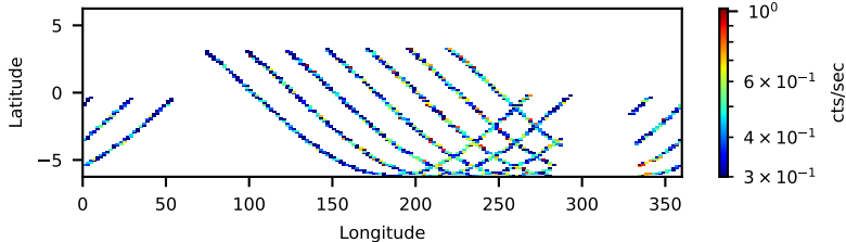
60802013004: 30 to 120 keV
