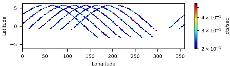
60802002028: 3 to 10 keV
