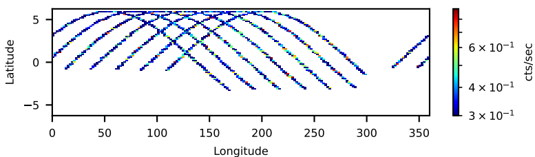
60802002028: 30 to 120 keV
