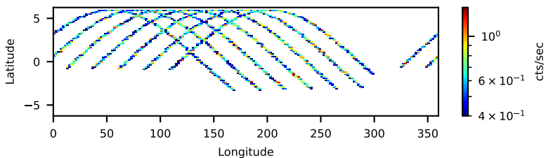
60802002028: 3 to 120 keV
