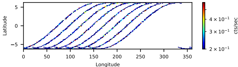
60802002016: 3 to 10 keV
