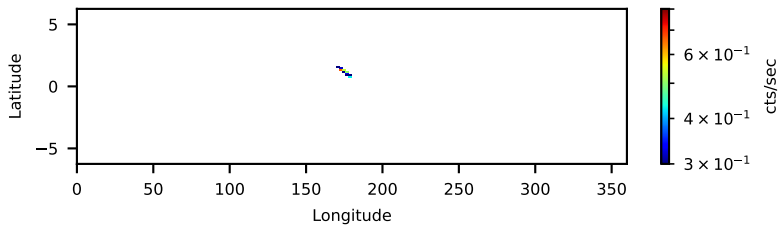
60802002003: 30 to 120 keV
