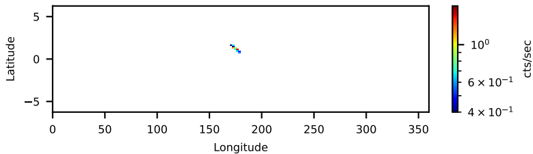
60802002003: 3 to 120 keV
