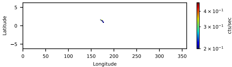
60802002003: 3 to 10 keV
