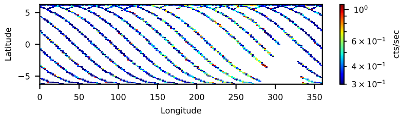
60801046002: 30 to 120 keV
