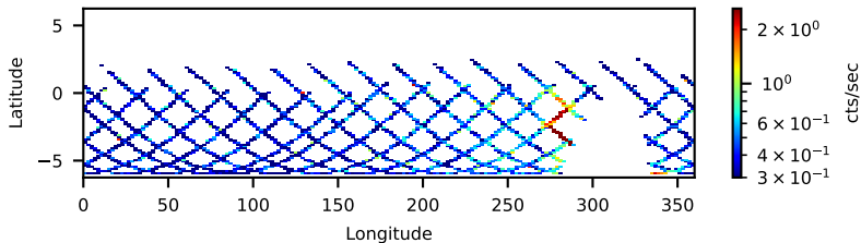
60801043002: 30 to 120 keV
