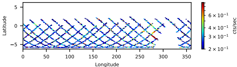
60801043002: 3 to 10 keV
