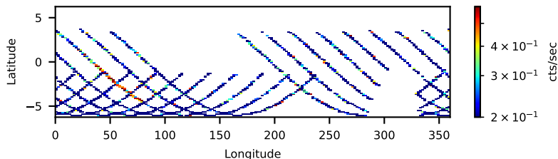
60801040002: 3 to 10 keV
