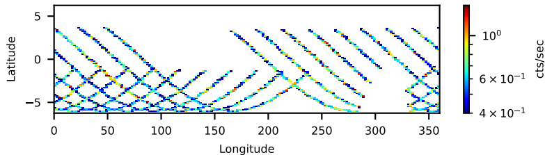
60801040002: 3 to 120 keV
