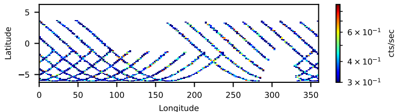
60801040002: 30 to 120 keV
