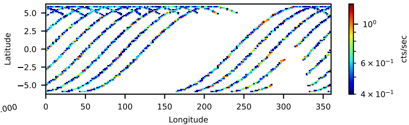
60801035002: 3 to 10 keV
