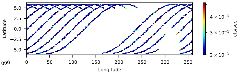
60801035002: 30 to 120 keV
