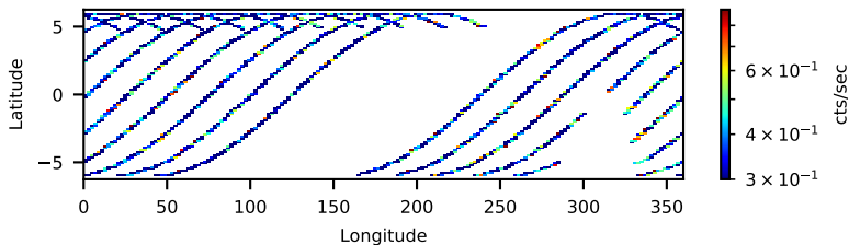
60801035002: 30 to 120 keV
