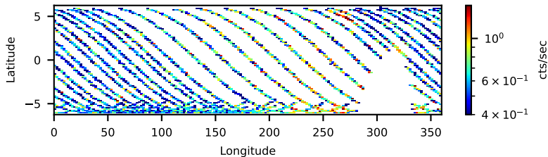
60801033004: 3 to 120 keV
