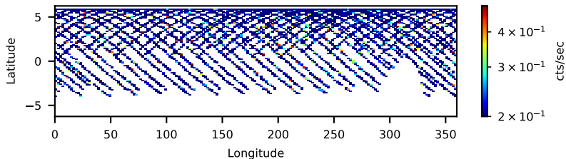
60801029004: 3 to 10 keV
