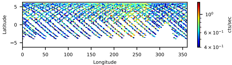
60801029004: 3 to 120 keV
