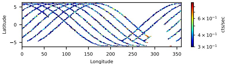
60801025004: 30 to 120 keV
