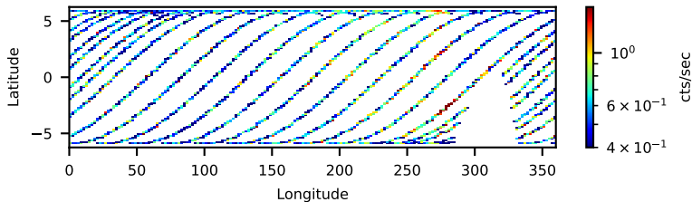
60801021002: 3 to 120 keV
