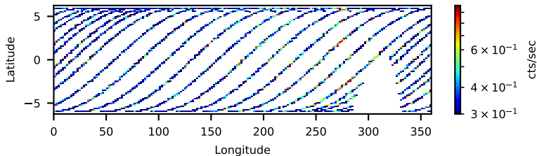
60801021002: 30 to 120 keV
