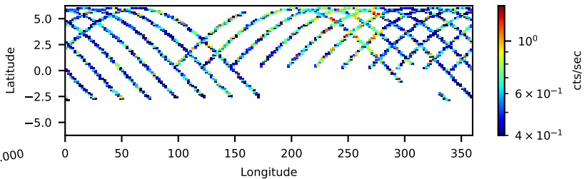
60801015006: 3 to 10 keV
