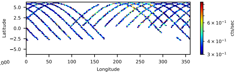
60801015006: 30 to 120 keV
