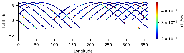
60801015006: 3 to 10 keV
