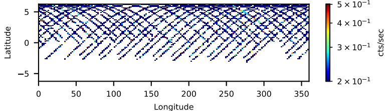
60801008002: 3 to 10 keV
