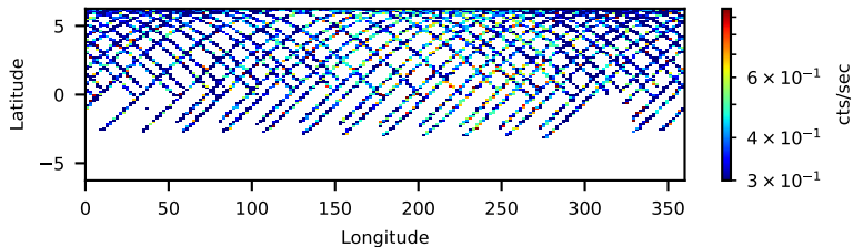
60801008002: 30 to 120 keV
