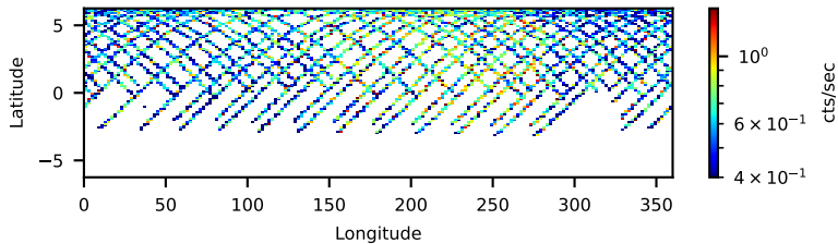
60801008002: 3 to 120 keV
