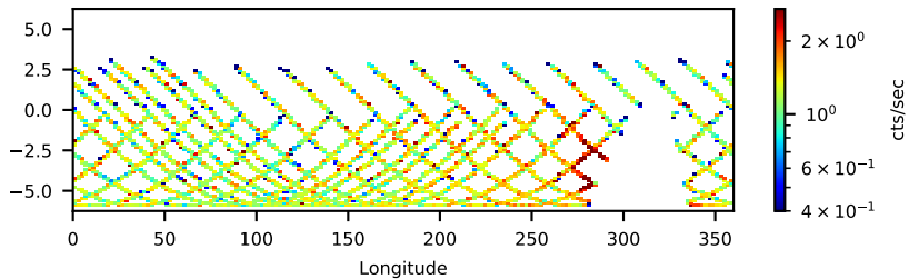
60801007002: 3 to 10 keV
