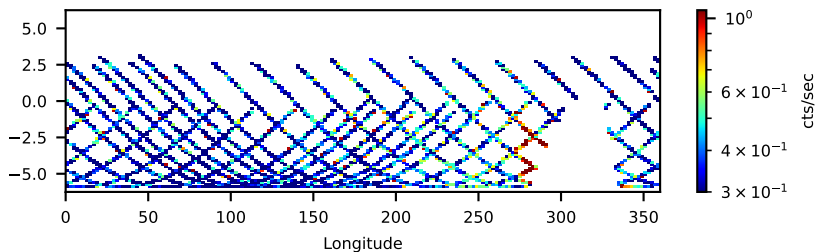
60801007002: 30 to 120 keV
