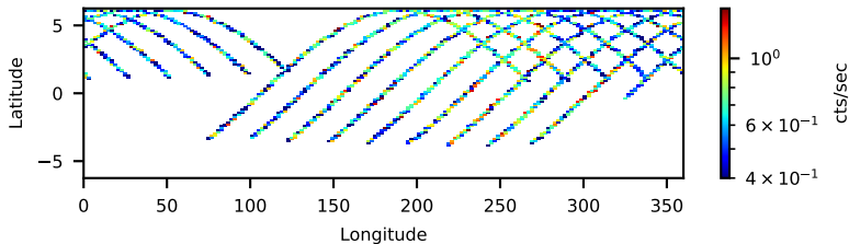
60801004002: 3 to 120 keV
