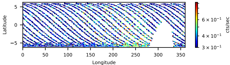
60763001002: 30 to 120 keV
