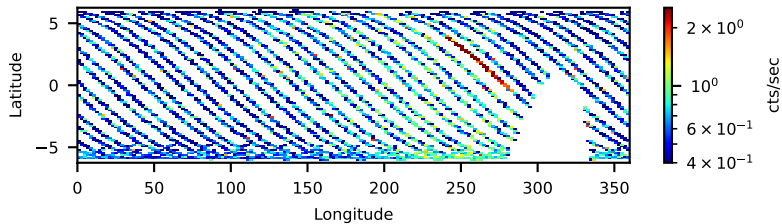
60763001002: 3 to 120 keV
