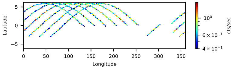
60761013002: 3 to 120 keV
