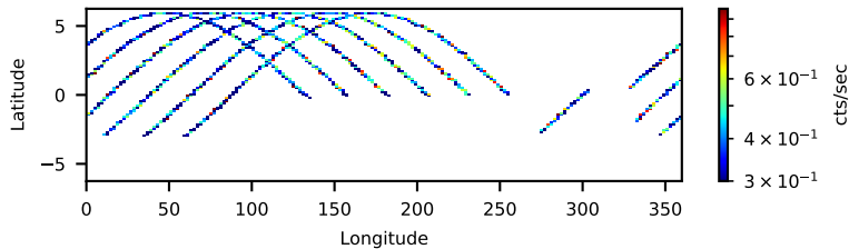
60761013002: 30 to 120 keV
