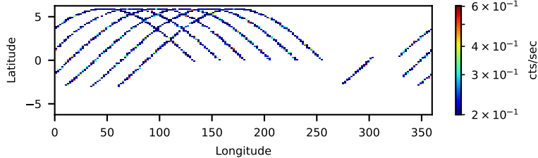
60761013002: 3 to 10 keV
