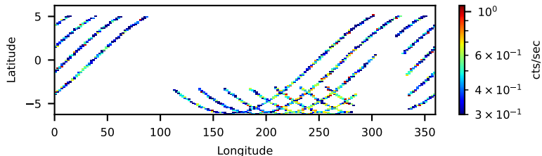
60761011002: 30 to 120 keV
