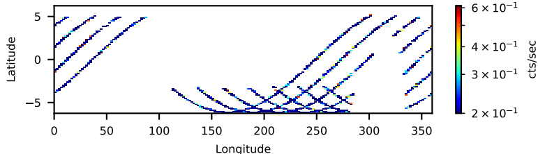
60761011002: 3 to 10 keV
