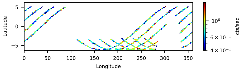
60761011002: 3 to 120 keV
