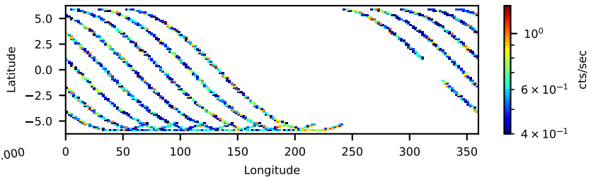
60761010002: 3 to 10 keV
