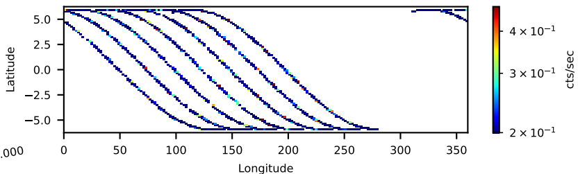
60761008002: 30 to 120 keV
