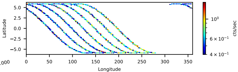
60761008002: 3 to 10 keV
