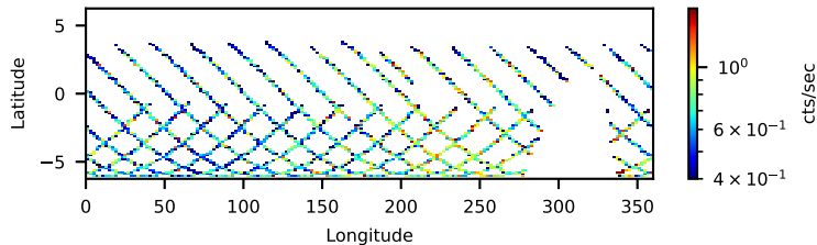
60702058004: 3 to 120 keV
