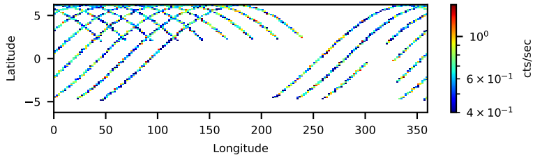
60702053006: 3 to 120 keV
