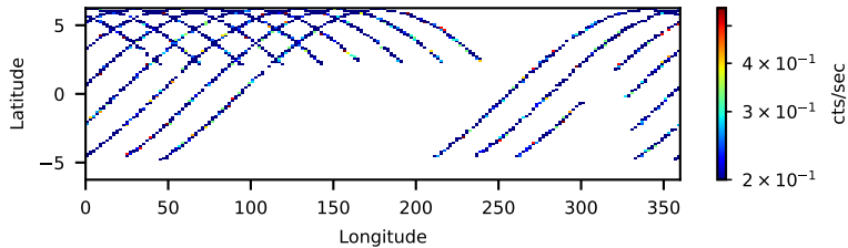
60702053006: 3 to 10 keV
