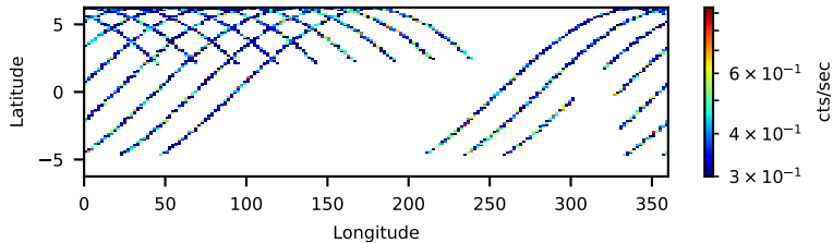
60702053006: 30 to 120 keV
