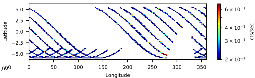
60702052004: 30 to 120 keV
