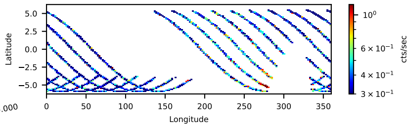
60702052004: 30 to 120 keV
