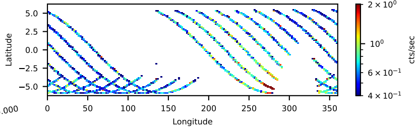
60702052004: 3 to 10 keV
