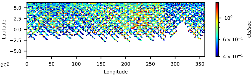
60701064006: 3 to 10 keV
