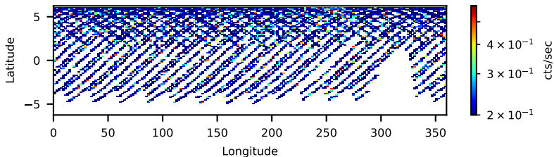
60701064002: 3 to 10 keV
