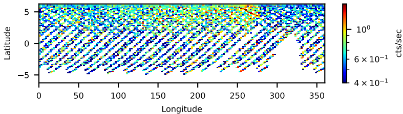
60701064002: 3 to 120 keV
