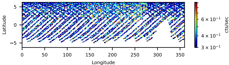
60701064002: 30 to 120 keV
