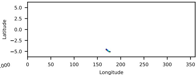
60701063003: 3 to 10 keV
