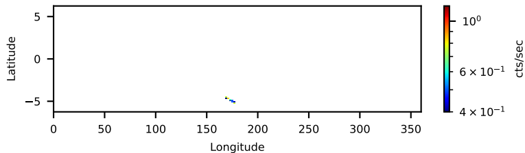
60701063003: 3 to 120 keV
