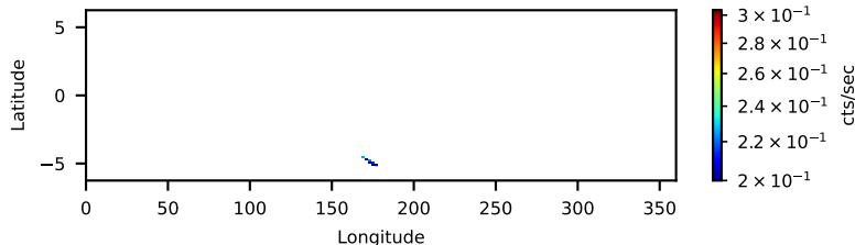
60701063003: 3 to 10 keV
