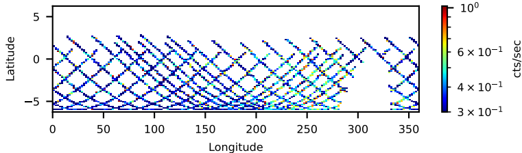
60701049002: 30 to 120 keV
