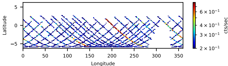
60701049002: 3 to 10 keV
