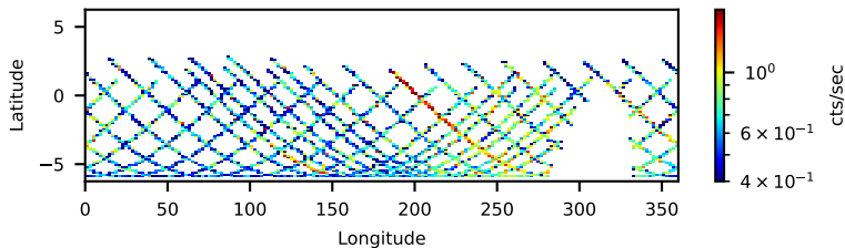
60701049002: 3 to 120 keV
