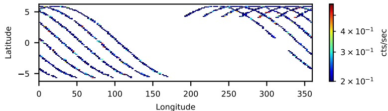
60701039002: 3 to 10 keV
