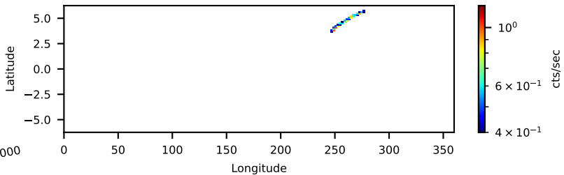
60701037001: 3 to 10 keV
