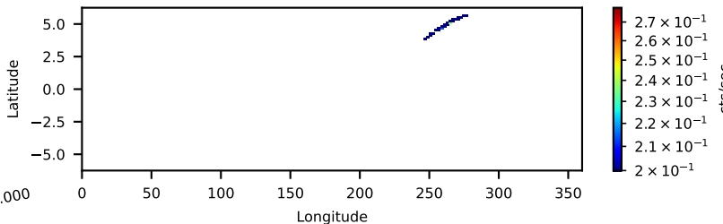
60701037001: 30 to 120 keV
