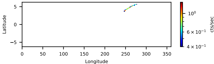
60701037001: 3 to 120 keV
