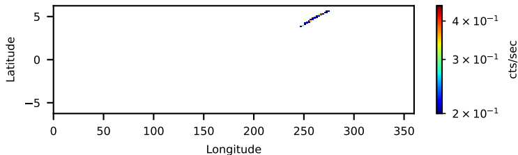
60701037001: 3 to 10 keV
