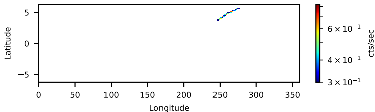
60701037001: 30 to 120 keV
