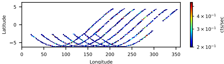
60701034002: 3 to 10 keV
