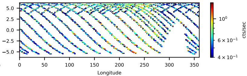
60701029002: 3 to 10 keV
