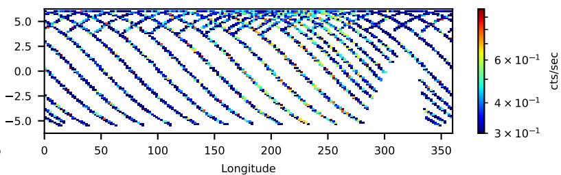
60701029002: 30 to 120 keV
