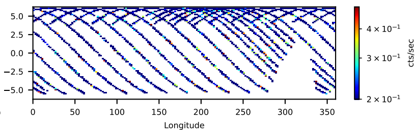
60701029002: 3 to 10 keV
