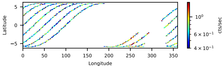
60701021002: 3 to 120 keV
