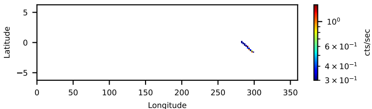
60701015001: 30 to 120 keV
