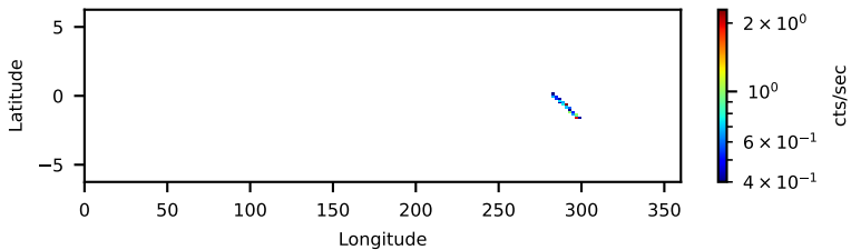
60701015001: 3 to 120 keV
