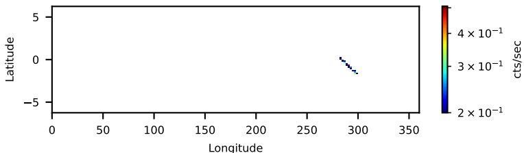
60701015001: 3 to 10 keV
